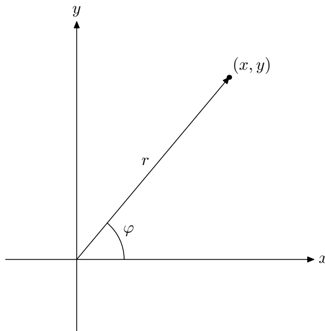
Abbildung 5.1: Ebene Polarkoordinaten
