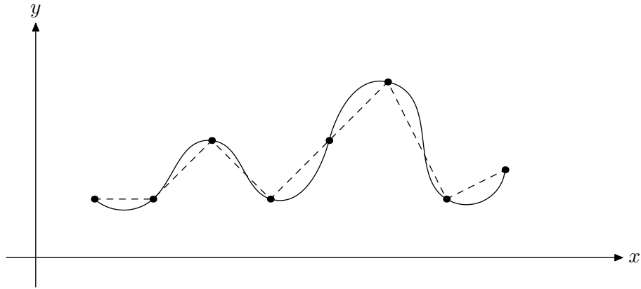
Abbildung 4.3: Bogenlänge
