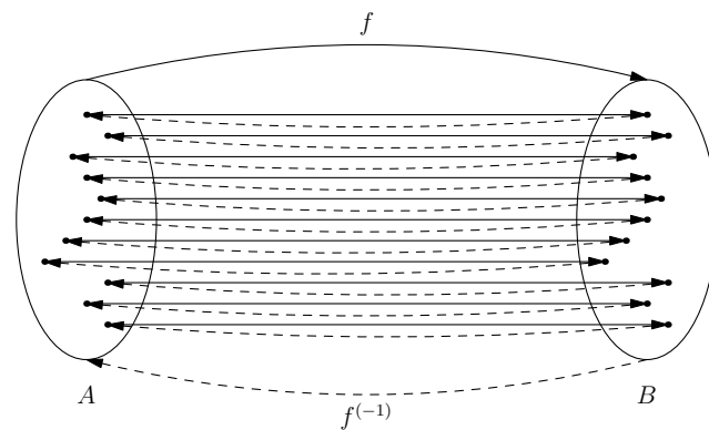
Abbildung 0.4: Eine bijektive Abbildung
