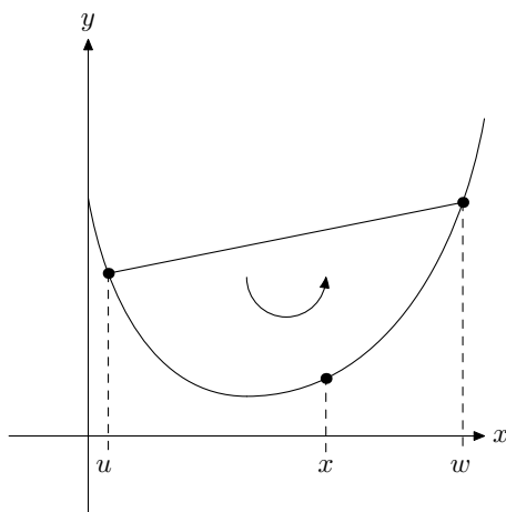
Abbildung 3.6: Graph einer konvexen Funktion
